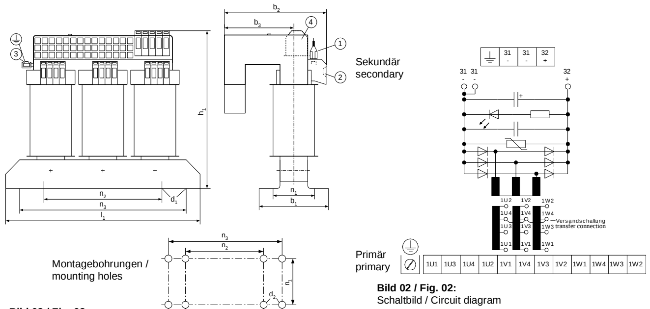
Bild 03 / Fig. 03: Raumbedarfsmaße und Anschlüsse / Space requirement dimensions of Terminals
