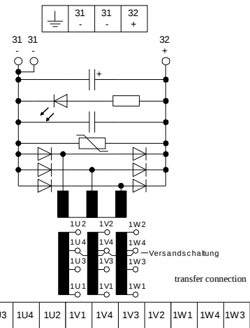
Bild 02 / Fig. 02: Schaltbild / Circuit diagram
