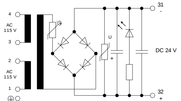
Bild 02 / Fig. 02: Schaltbild / Circuit diagram
