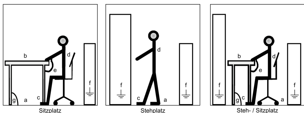
Bild 1-1 EGB-Schutzmaßnahmen
