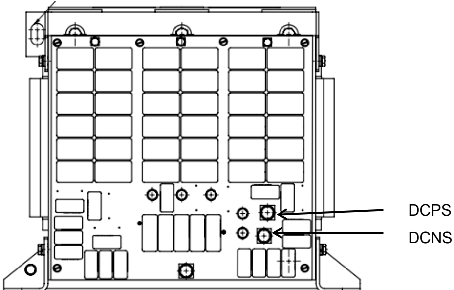
Bild 4-3 Kundenanschluss du/dt-Filter TEF1203-0JB
