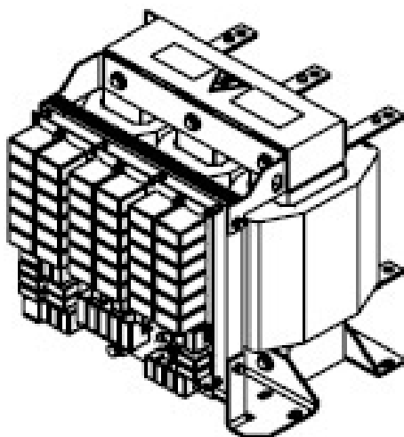
Bild 4-5 Anschlussstellenübersicht du/dt-Filter TEF1203-0LB
