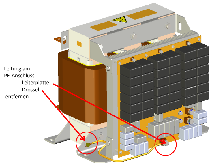
Bild 4-8 Verbindungsleitung zu den Kondensatoren des Gleichtaktfilters
