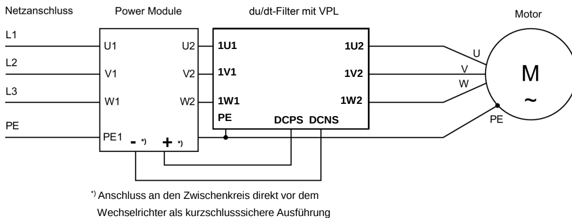
Bild 4-7 Anschluss-Übersicht
