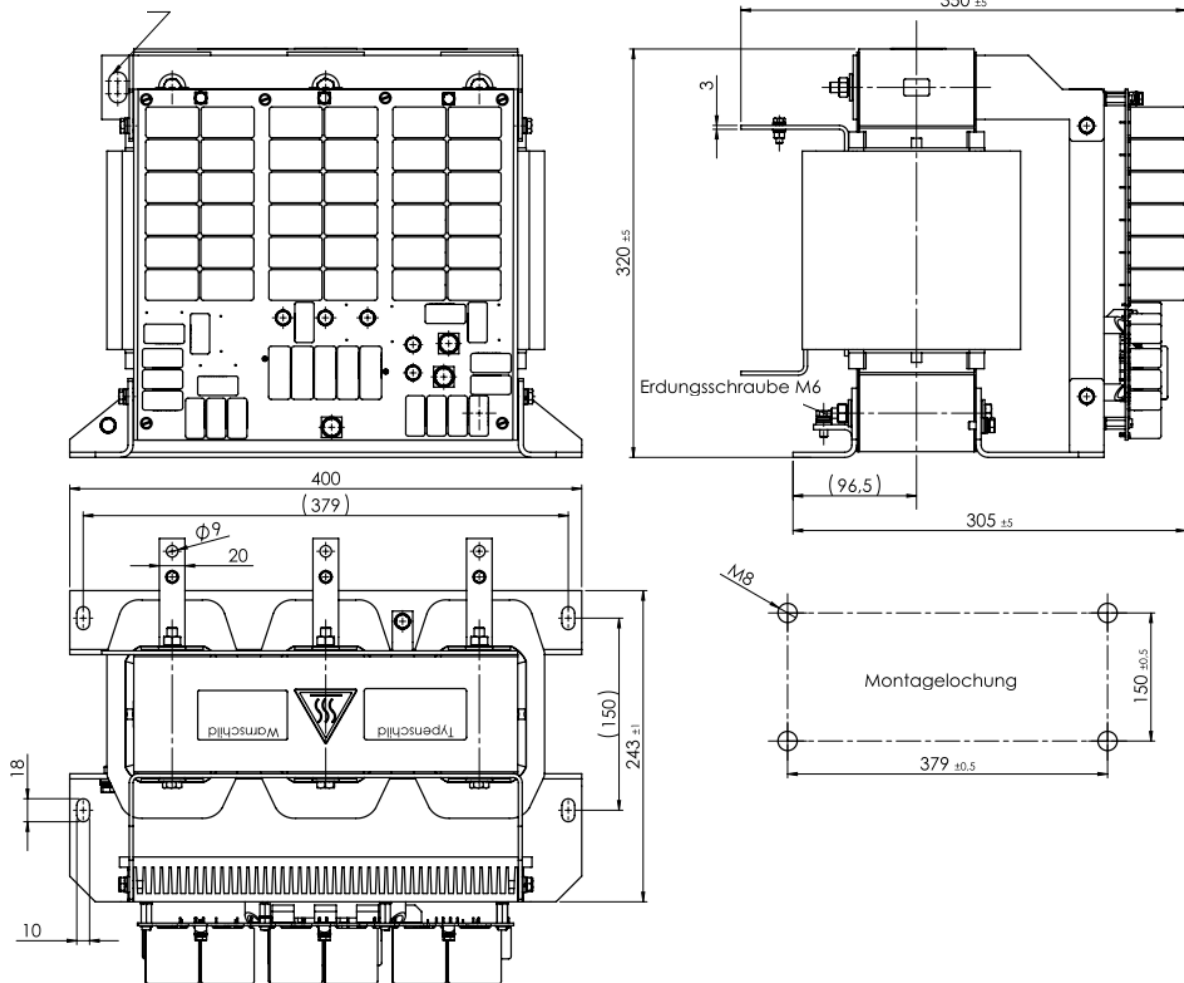
Bild 3-4 Maßblatt du/dt-Filter MTZEF051-24
