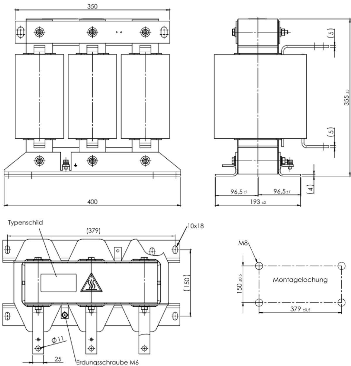
Bild 3-7 Maßblatt Ausgangsdrössel MTZEU182-117
