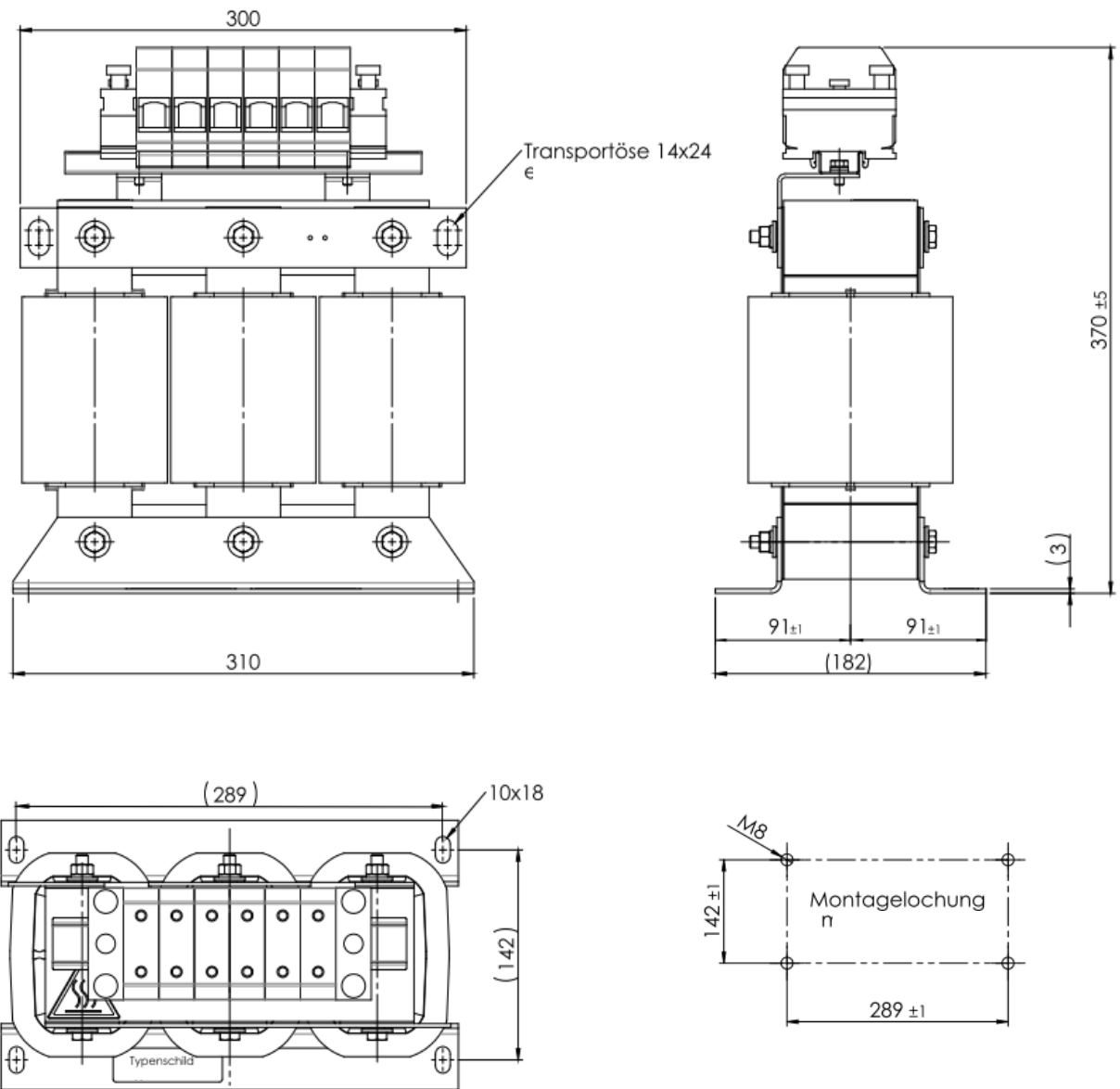
Bild 3-5 Maßblatt Ausgangsdrossel MTZEU129-114
