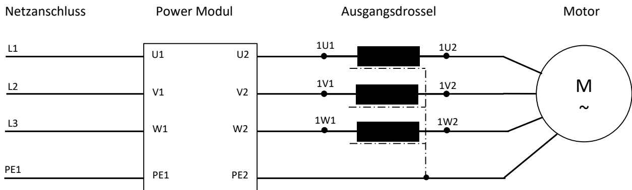
Bild 4-5 Anschluss-Übersicht
