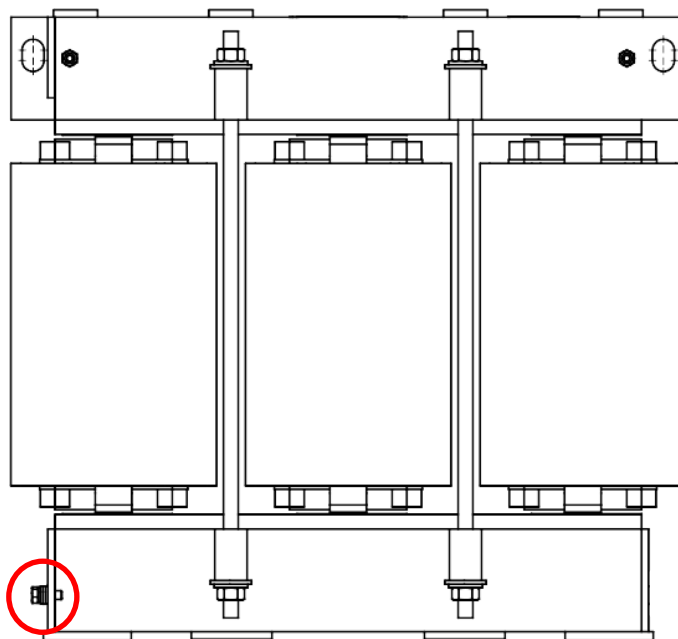
Bild 4-4 Anschlussstellenübersicht Ausgangsdrossel TEU4732-0FA00-0BA0
