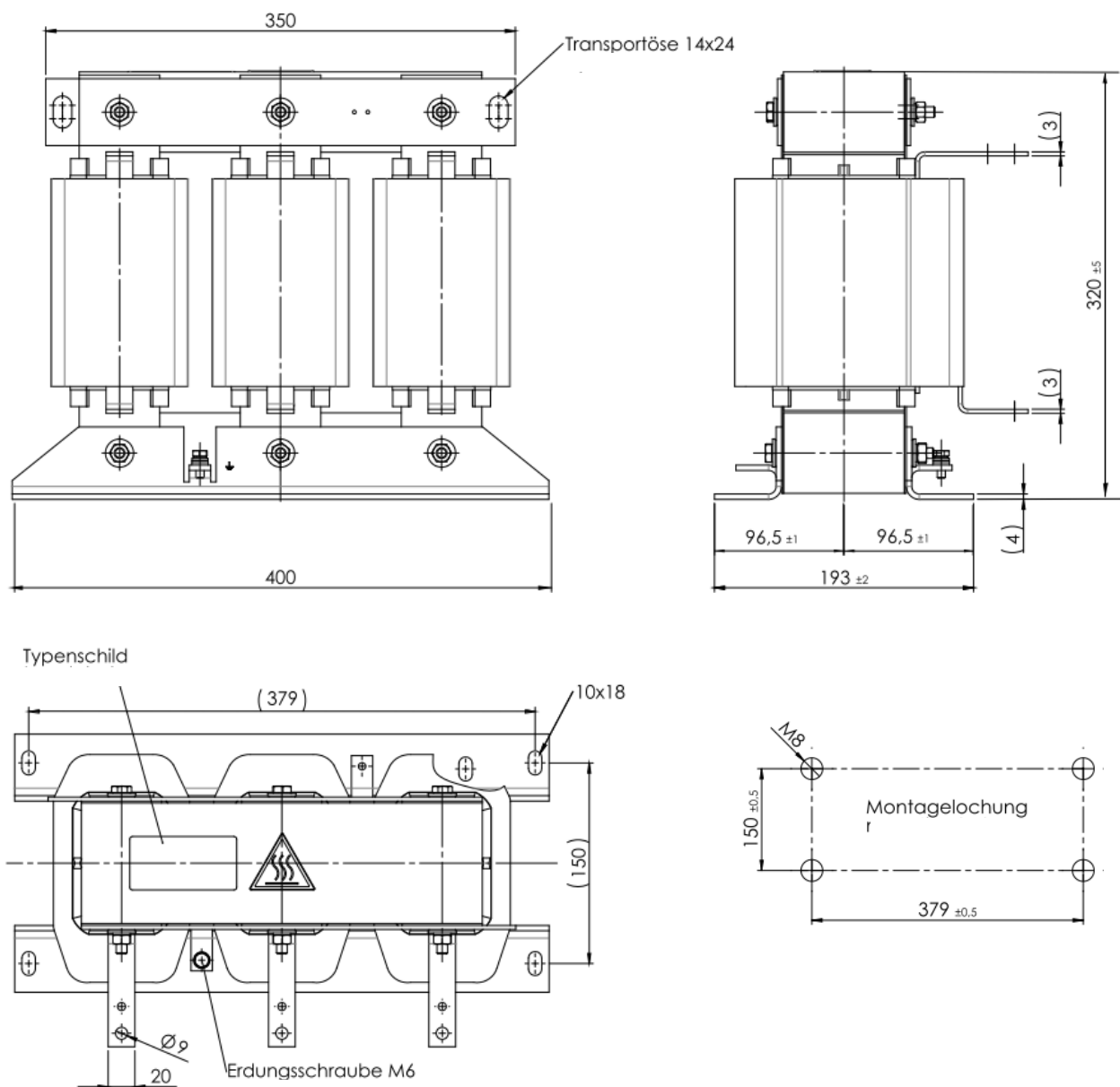
Bild 3-6 Maßblatt Ausgangsdrössel MTZEU182-116
