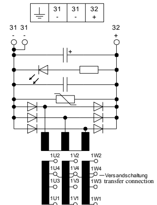
Bild 02 / Fig. 02: Schaltbild / Circuit diagram
